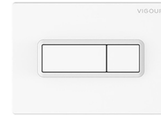
BETÄTIGUNGSPLATTE seidenmatt, Breite: 205 mm, Höhe: 145 mm
