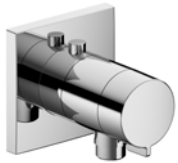
BRAUSETHERMOSTAT aus Messing / verchromt, eckig, Breite: 90 mm, Höhe: 90 mm, Ausladung: 100 mm
