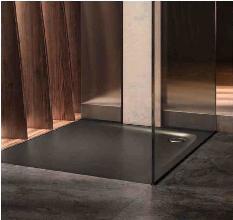
DUSCHFLÄCHE aus Kaldewei Stahl-Email, Länge: 800 – 1.800 mm, Breite: 700 – 1.200 mm, Tiefe: 25 – 51 mm
